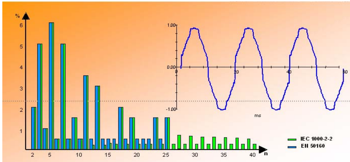
Abb. 1.2 Vergleich der Verträglichkeitspegel der Spannungsoberschwingungen nach EN 61000-2-2 und EN 50160 mit Darstellung der entsprechenden Kurvenform 1
